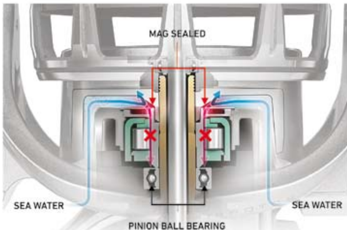
Vergleich von Rollen mit MAG SEALED und ohne. Quelle DAIWA Intern - Service-Abt.
