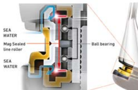
Rollen mit MAG SEALED Schnurlaufröllchen und ohne. Quelle DAIWA Intern - Service-Abt.
